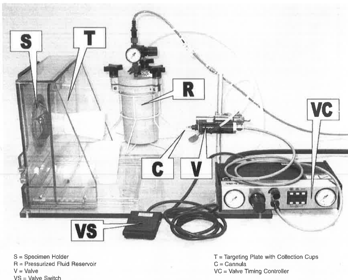
FIG. 1 (a) Test Apparatus
