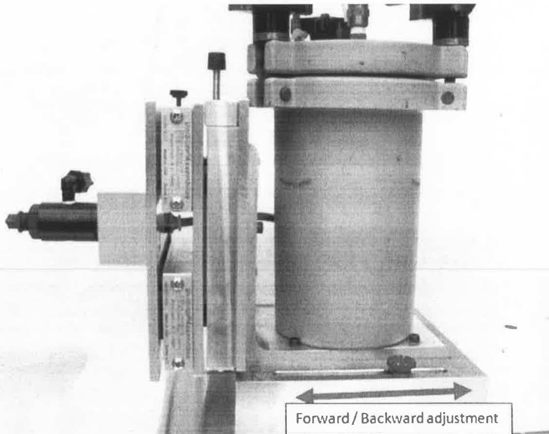
FIG. 1 (d) Forward and Backward Adjustment (continued)
